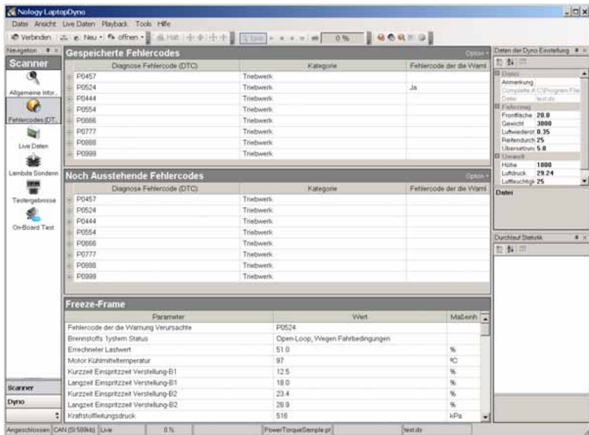
Figure 3: Fehlercodes Fenster
